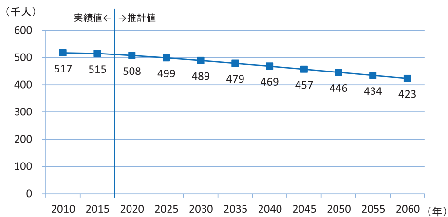
図表VI-18 人口ビジョンにおける人口将来展望
