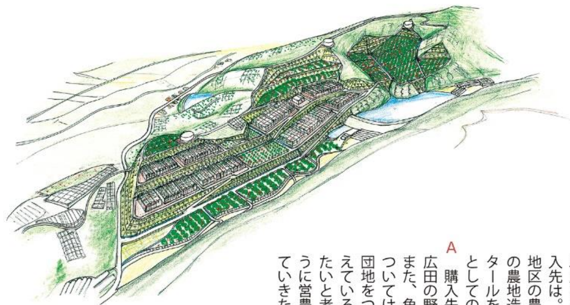
農地中間管理機構関連農地整備事業 砥部地区 整備構想図
