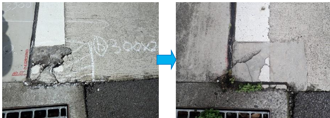
図３ 断面修復（コンクリート舗装）
